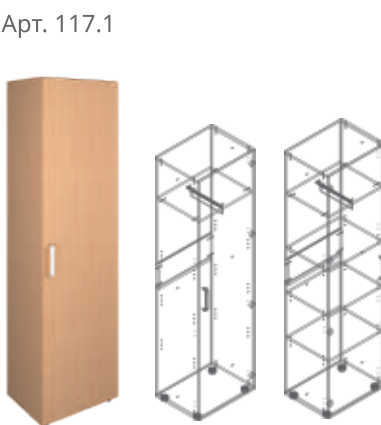
Шкаф для одежды 1-дверный (500x370x1872)
